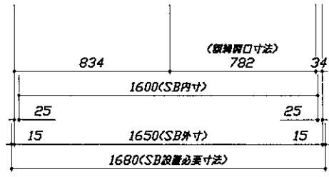
<平面図>
