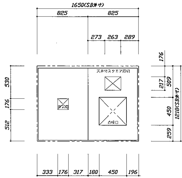
<天井伏図>
