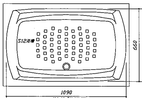
<浴槽詳細図>
