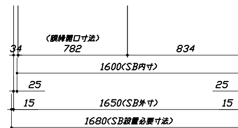
<平面図>
