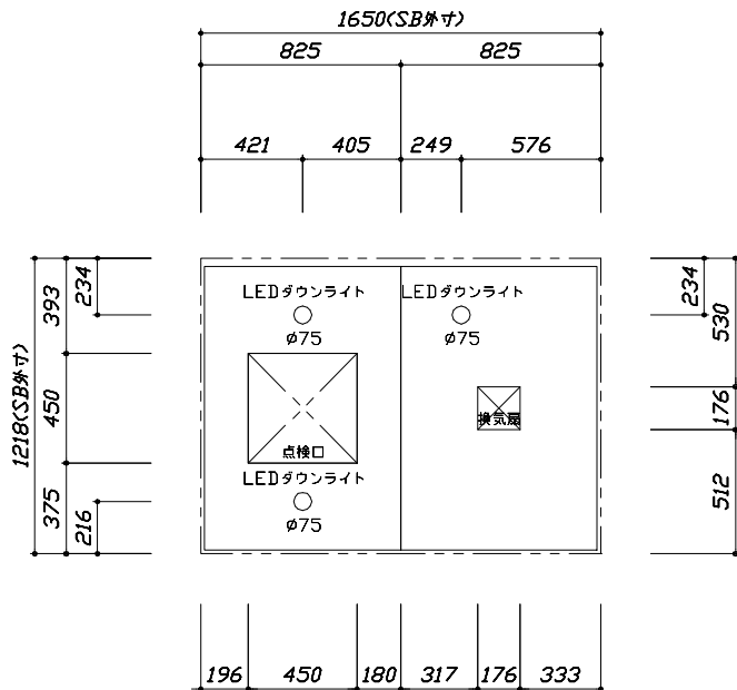
<天井伏図>
