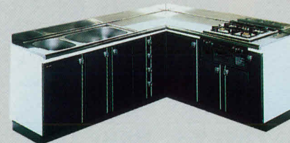
開口210cm CKLW-210GB (左・右水槽) 2,100×1,800×819mm ¥423,000 ●写真の商品は左水槽です。
