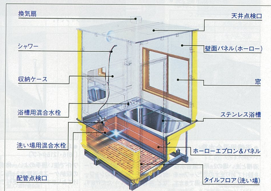
● ステンレスハニカム構造(タイル下)
