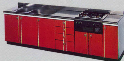
開口270cm CKW-270GF (左・右水槽) 2,698×800×819mm ¥338,000 ●写真の商品は左水槽です。
