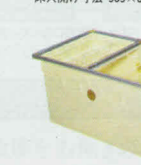
開口90cm UA-90 919×616×458mm 網トレイ① ¥21,500 床穴開け寸法 909×606mm
