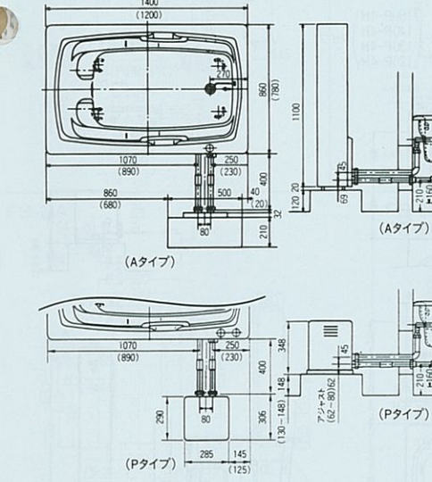
配管仕様3 FUB-1403Hタイプ・FUB-140P-3Hタイプ(接続配管:ハイカンB-40LS使用) (1203H) (120P-3H)
