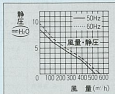
●VF-60特性
