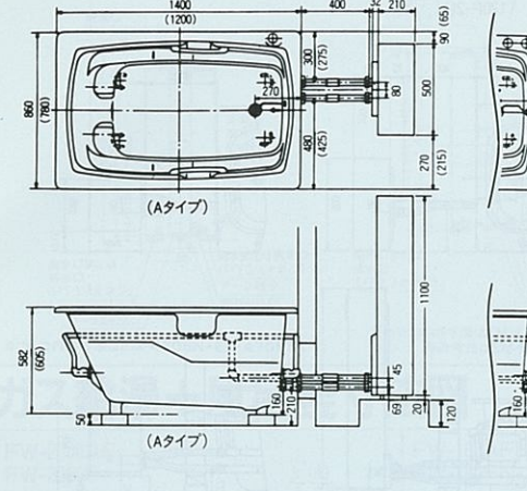
配管仕様3 FUB-1403Hタイプ・FUB-140P-3Hタイプ(接続配管:ハイカンB-40LS使用) (1203H) (120P-3H)
