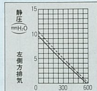
●VP-60特性
