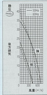
●VB-60・75特性
