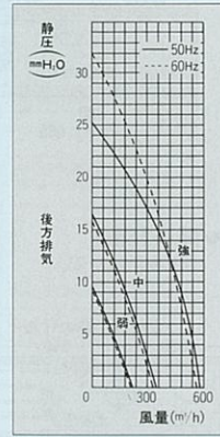
●VCN-60特性
