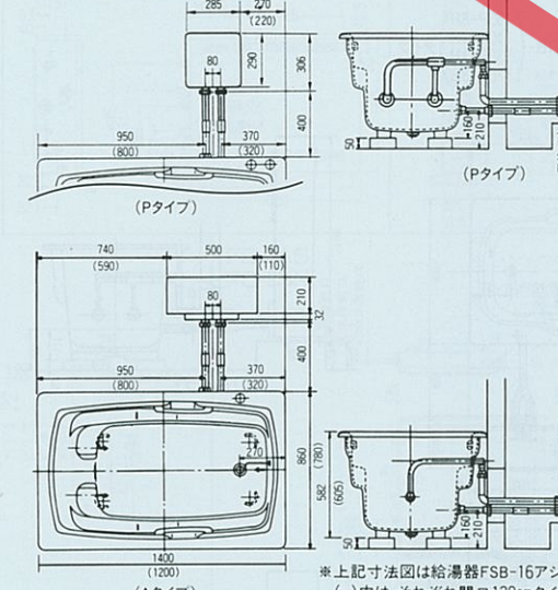
配管仕様4 FUB-1404Hタイプ・FUB-140P-4Hタイプ(接続配管:ハイカンB-40LS使用) (1204H) (120P-4H)
