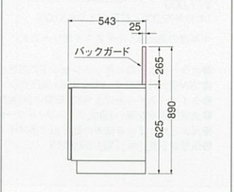
バックガード・ガス台セット図面
