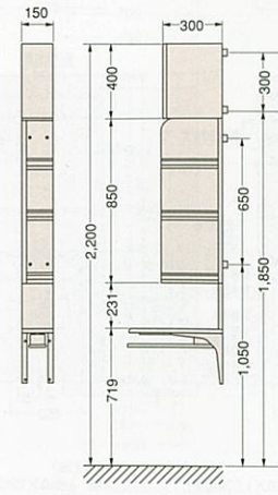
●SIC-15(タオルハンガー)
