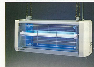
MTB-020 幅800×奥行303×高さ323mm 屋外用 (軒下用) 本体価格 ¥69,500
