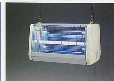
MTS-015 幅550×奥行320×高さ315mm 屋内用 本体価格 ¥39,000
