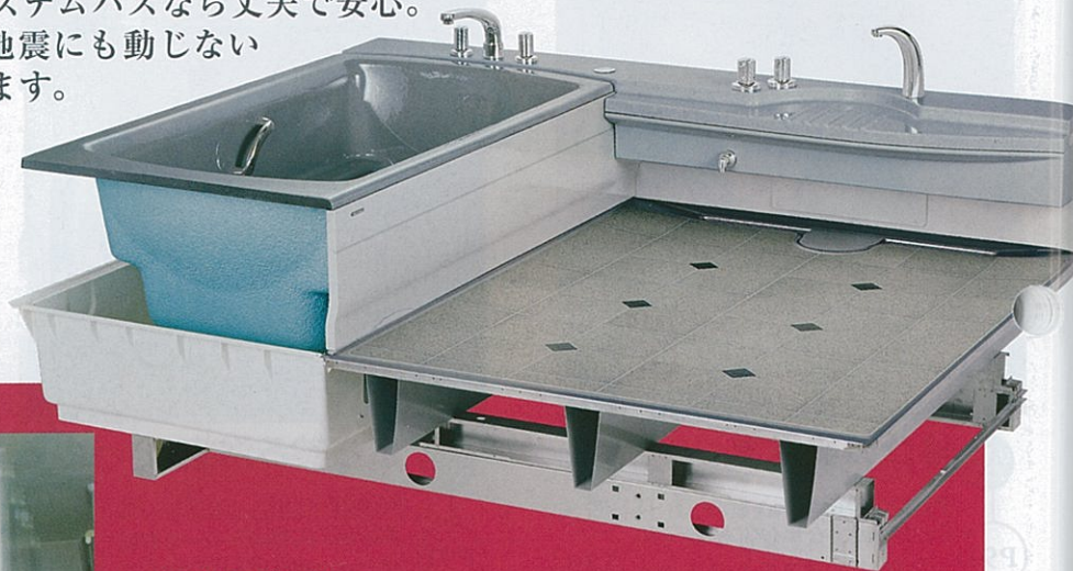
●システムバス ハーフユニット(下台部分) 写真はフレテンシアです。シリーズにより若干仕様異なります。
