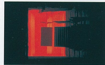
850℃の炉の中で金属とガラスを焼成して密着。
