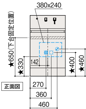
上面図
