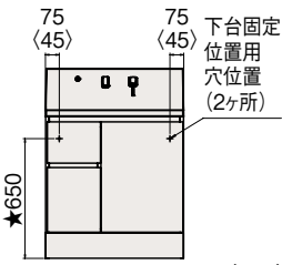
正面図
