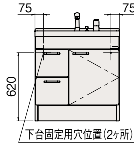
正面図
