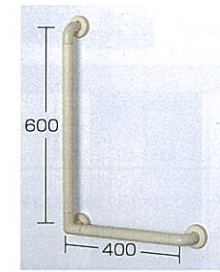
■L型 L型は左右兼用です。(写真はL型左方向での設置例)
