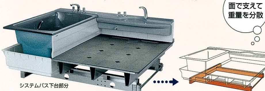
▲タカラシステムバス耐震実験の様子 (実験は、関西電力株式会社 電力技術研究所の振動実験装置を用いて行いました。) 実験条件 <実験状況> システムバスユニット単体での加振実験(振動台に架台を固定) <振動内容> 平均加速度: 800gal、振動周波数: 3~5Hz間で変移の振動(理論上の震度6強)を1分間加振
