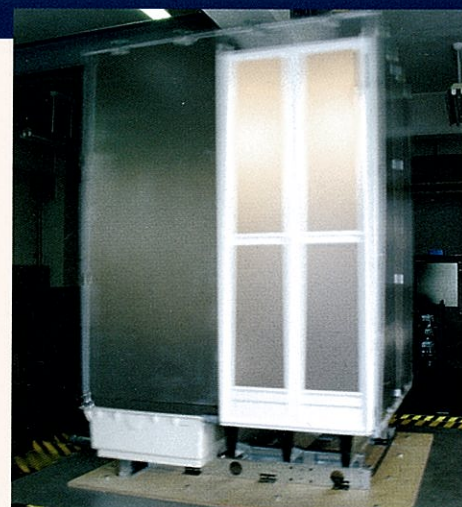
▲タカラシステムバス耐震実験の様子 (実験は、関西電力株式会社 電力技術研究所の振動実験装置を用いて行いました。) 実験条件 <実験状況> システムバスユニット単体での加振実験(振動台に架台を固定) <振動内容> 平均加速度: 800gal、振動周波数: 3~5Hz間で変移の振動(理論上の震度6強)を1分間加振
