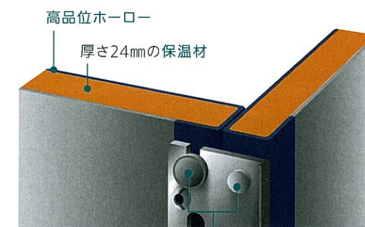
パネル同士を金具で固定
