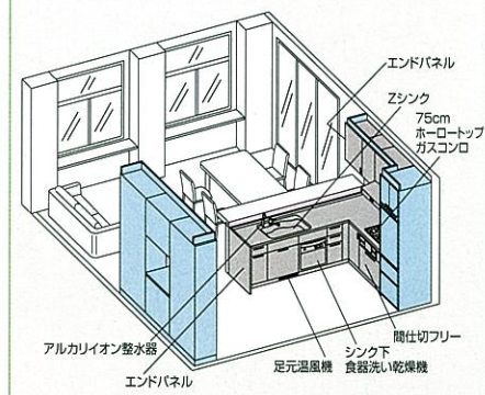
ベースキャビネット間口 シンク側255cm×加熱機器側180cm
