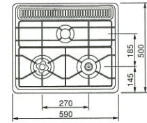
(イラストはBGC61-3PB)
