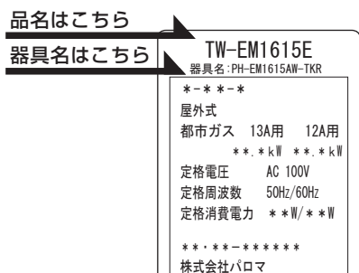
銘板 (例) 都市ガス用
