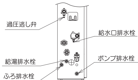
排水栓位置図
