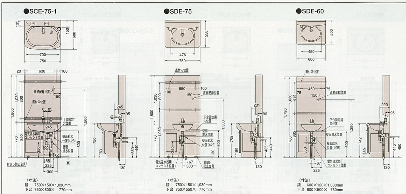
●電気温水器付洗面ユニット仕様表
