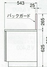
バックガード・ガス台セット図面
