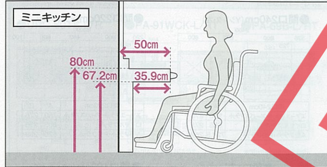
●ミニキッチンの膝まわり寸法
