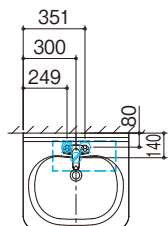
上面図
