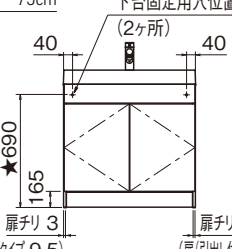
正面図
