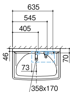
上面図
