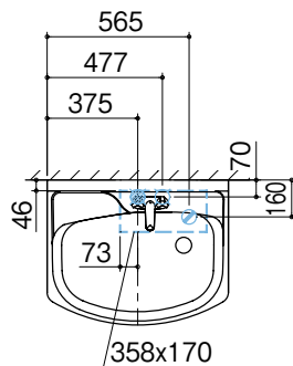
上面図
