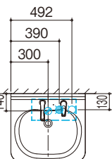
上面図
