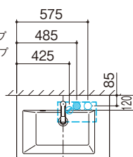
上面図
