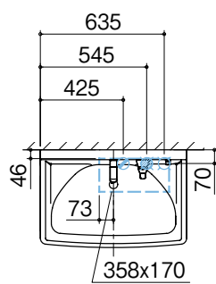
上面図
