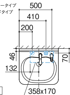
上面図
