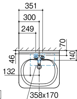
上面図
