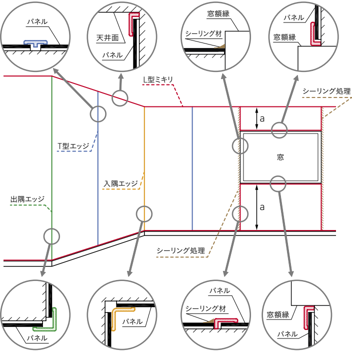
タテ設置図
