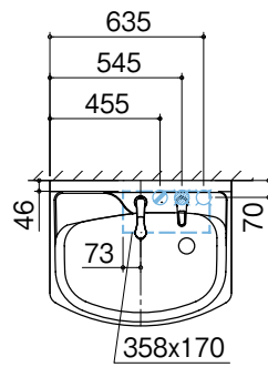
上面図
