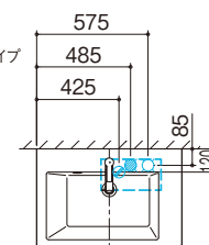
上面図
