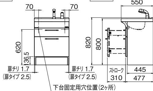
正面図
