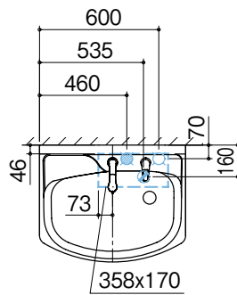
上面図
