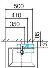
上面図
