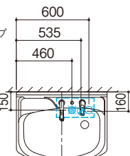
上面図
