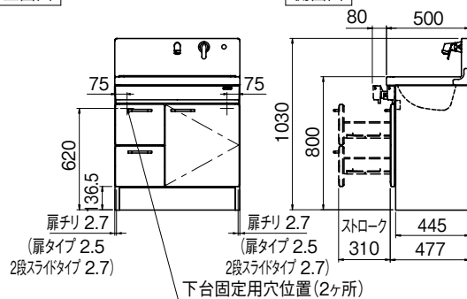
正面図
