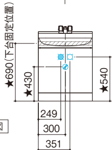
正面図
