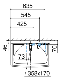
上面図
