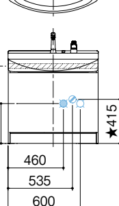
正面図
