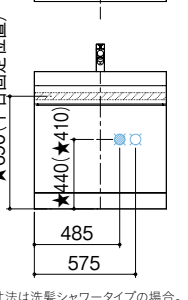
正面図
