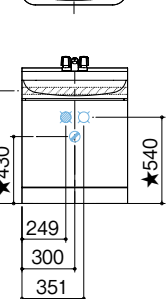
正面図
