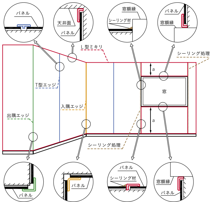
タテ設置図
