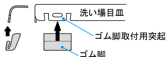
取付状態
