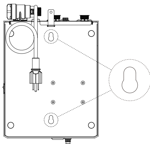
【背面図】
