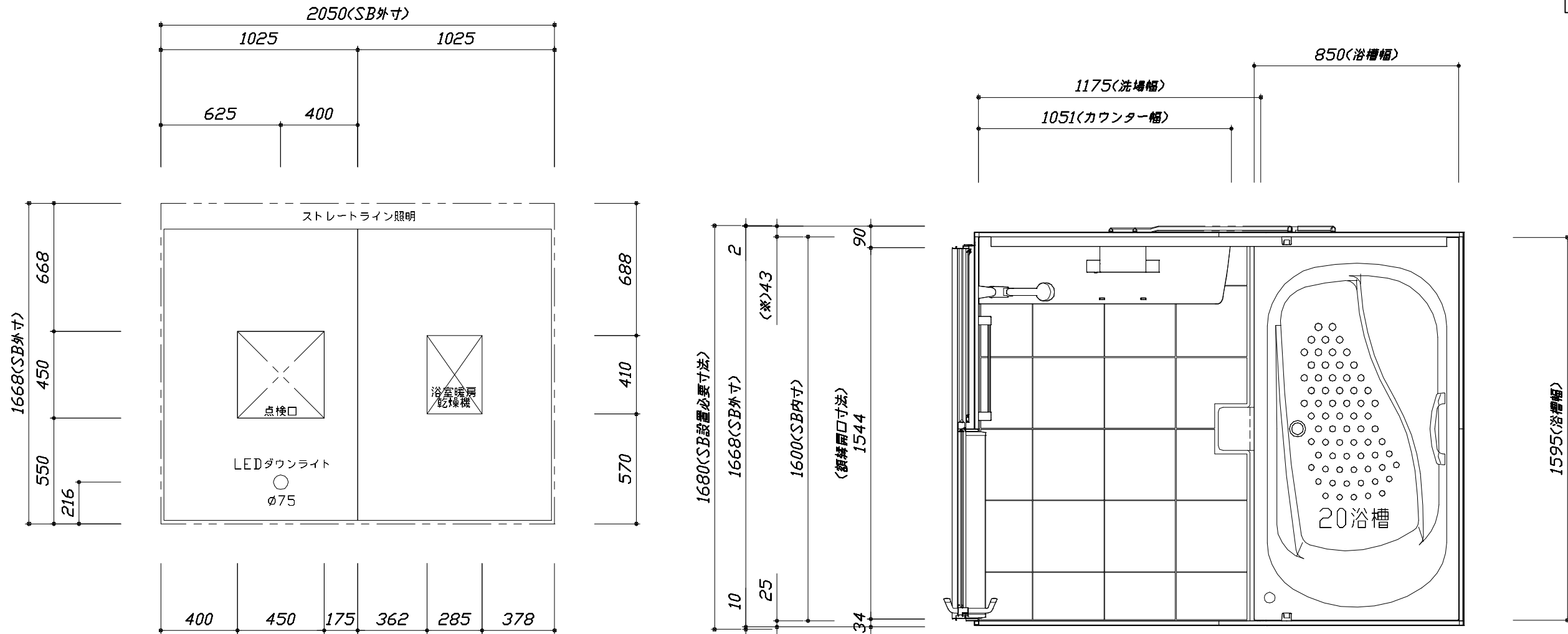
< 天井伏図 >
