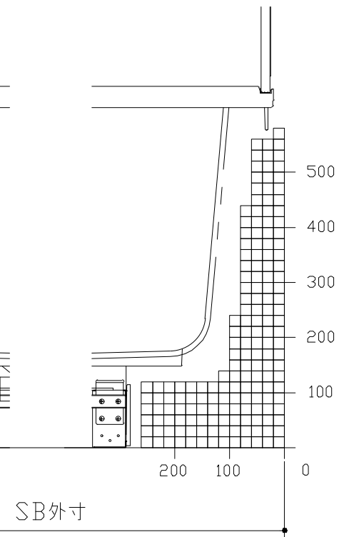
E矢視
