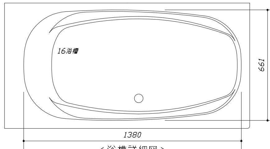
< 浴槽詳細図 >
