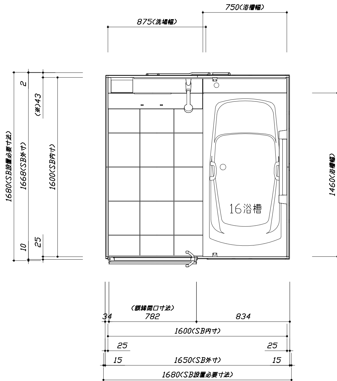
<平面図>
