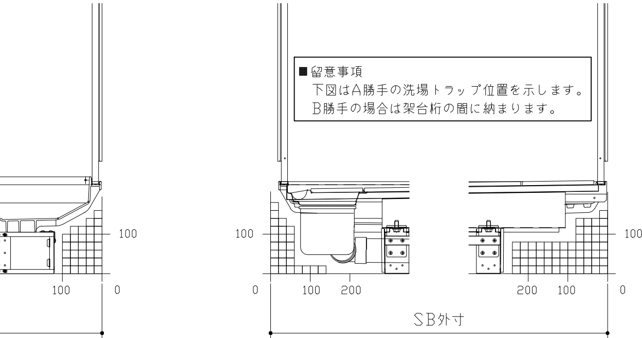
D矢視
