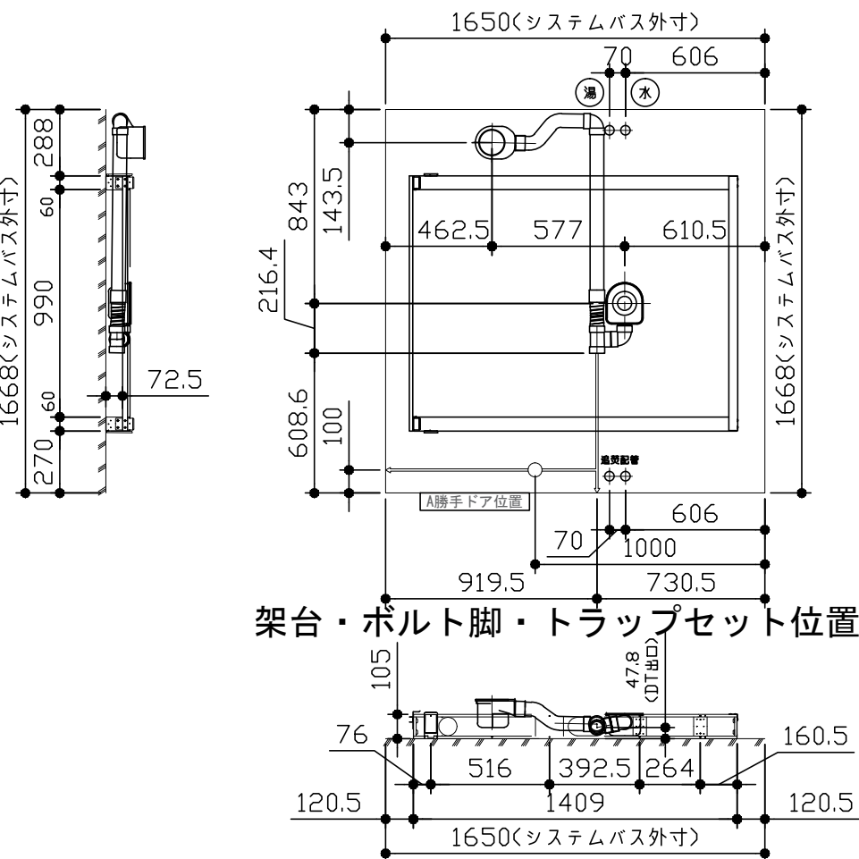
給水給湯管・追焚配管立上げ位置図
