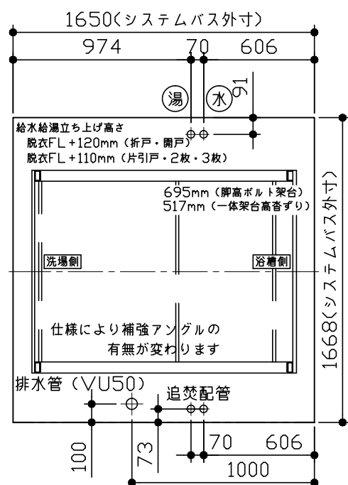
給水給湯管・追焚配管立上げ位置図
