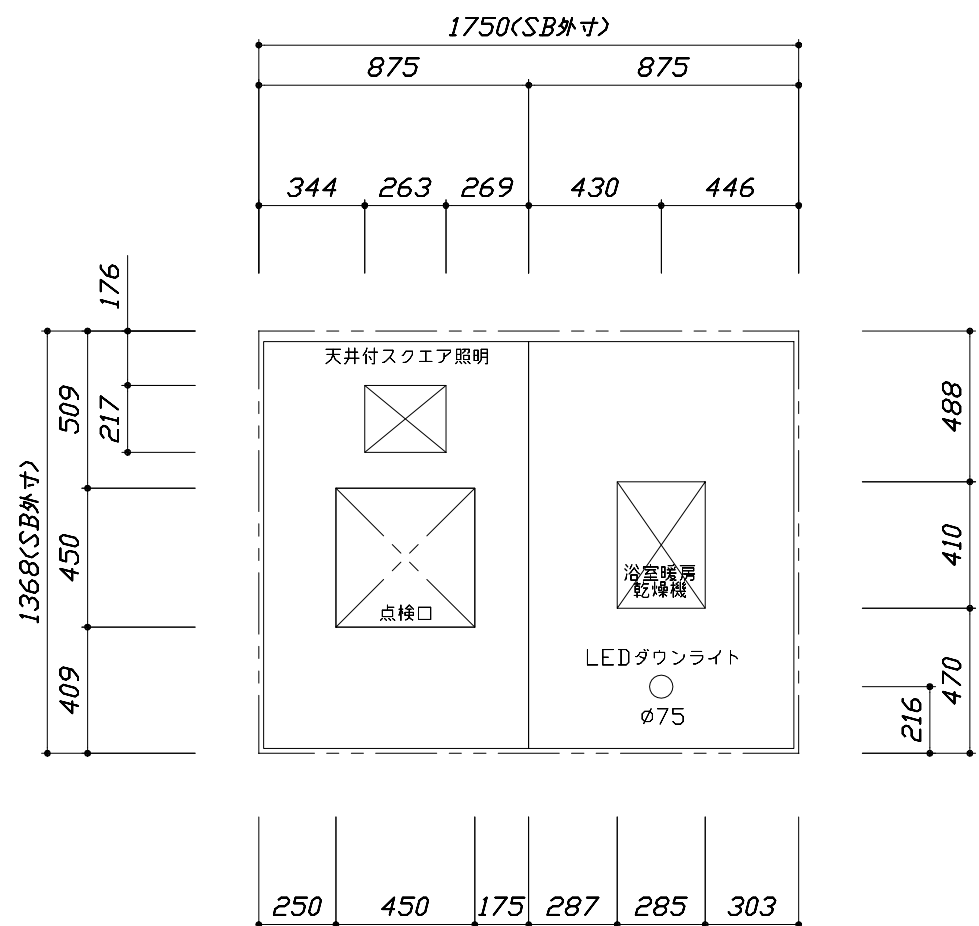
<天井伏図>
