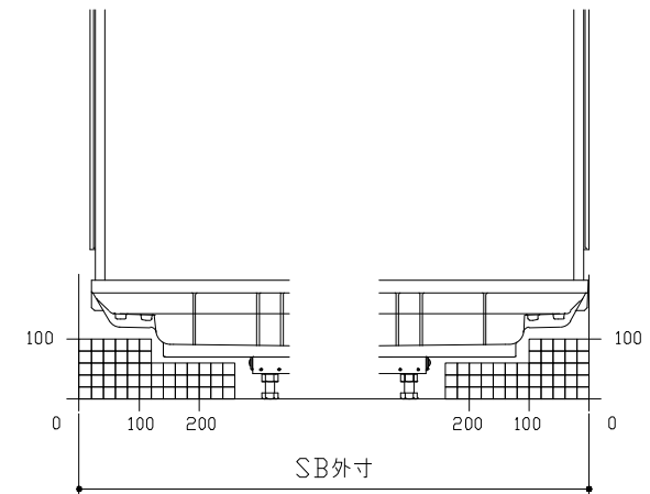
E矢視
