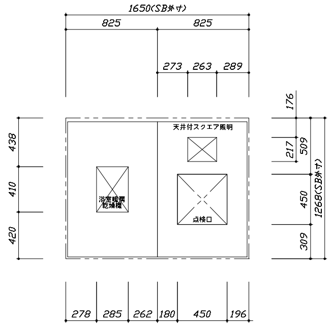
<天井伏図>
