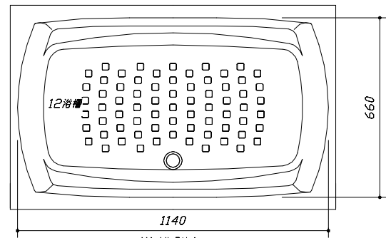
<浴槽詳細図>
