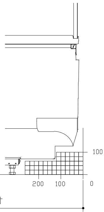
E矢視
