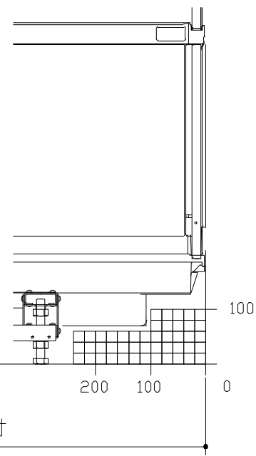
C矢視
