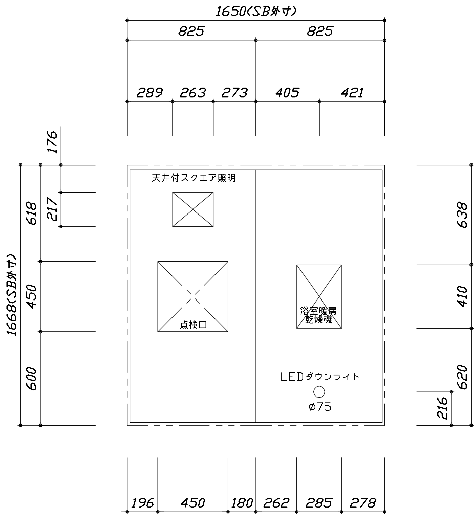
<天井伏図>
