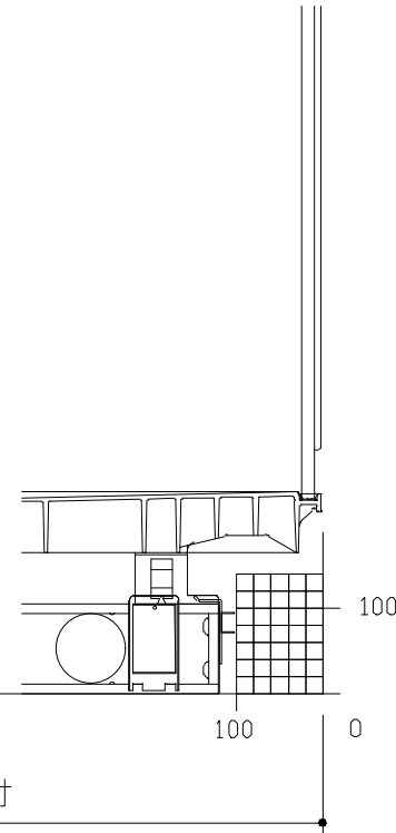
B矢視
