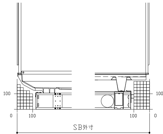
A矢視
