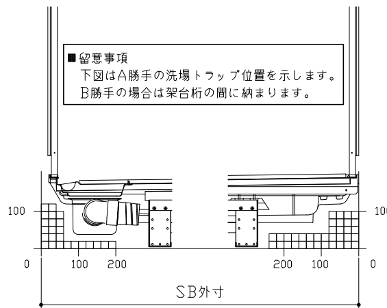
D矢視
