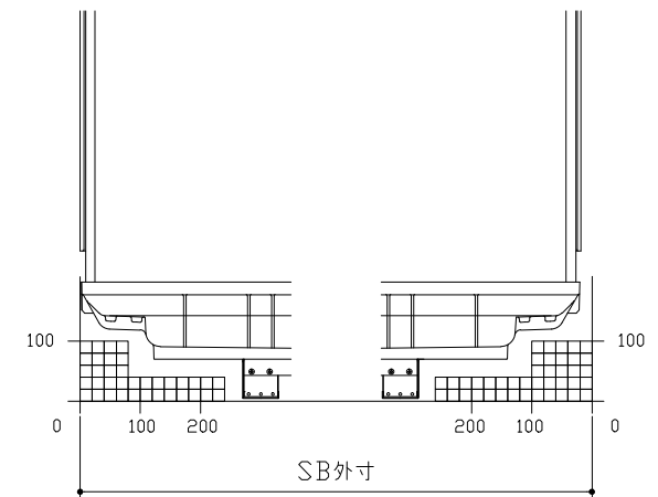
F矢視
