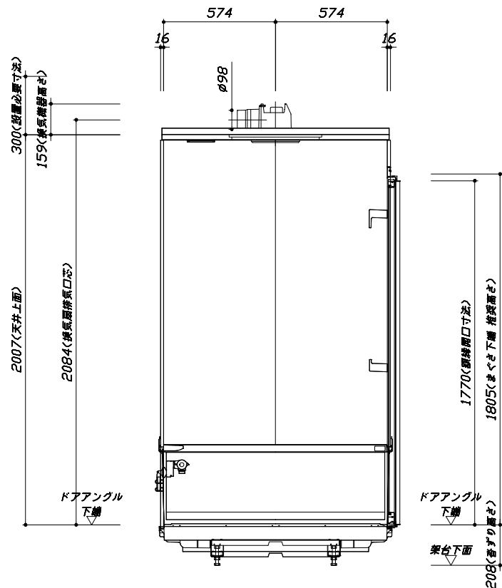
< 浴槽側面図 >
