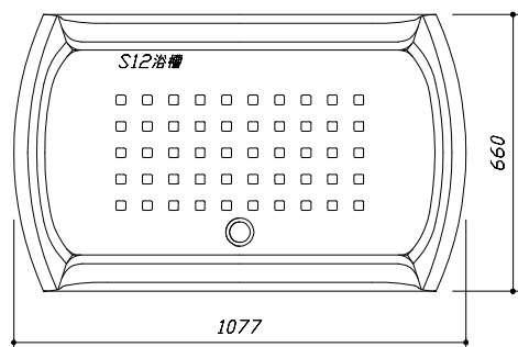
<浴槽詳細図>
