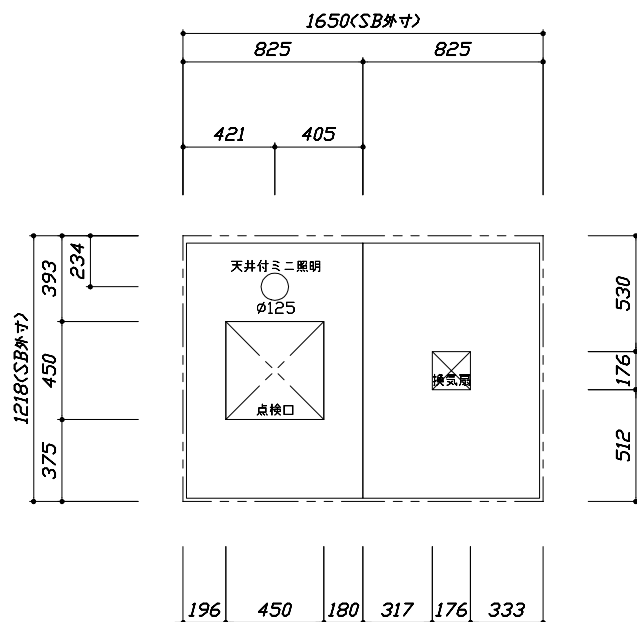
<天井伏図>
