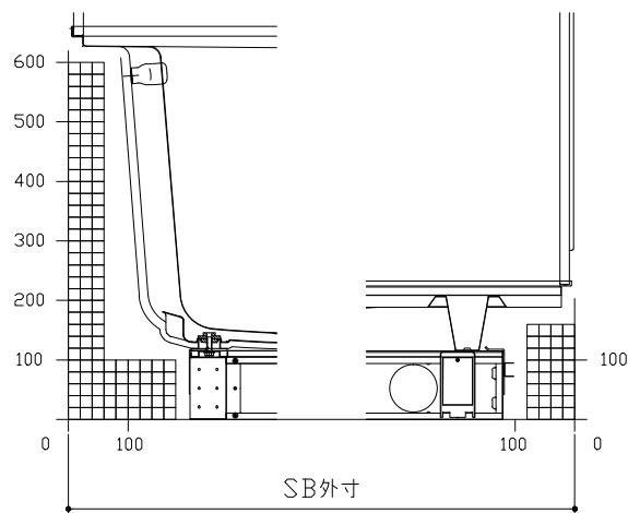
A矢視
