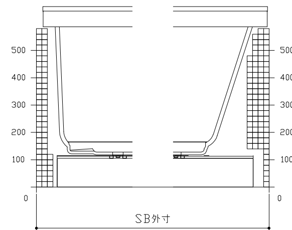
E矢視
