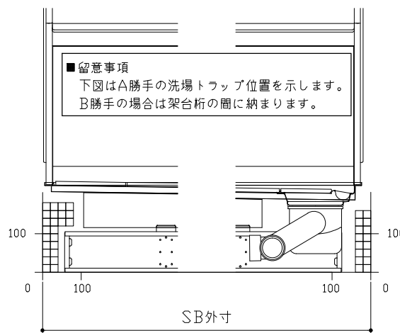
C矢視
