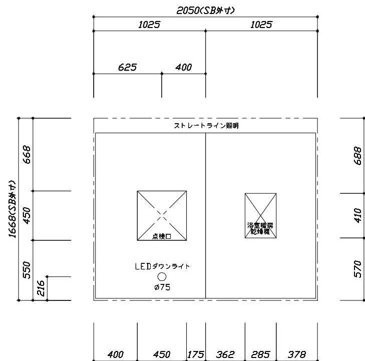
<天井伏図>
