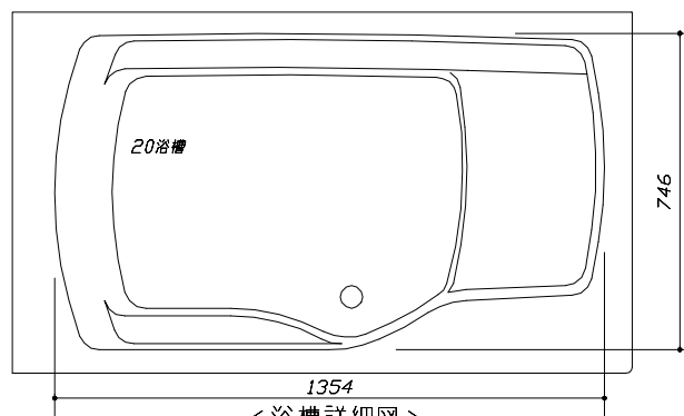
<浴槽詳細図>
