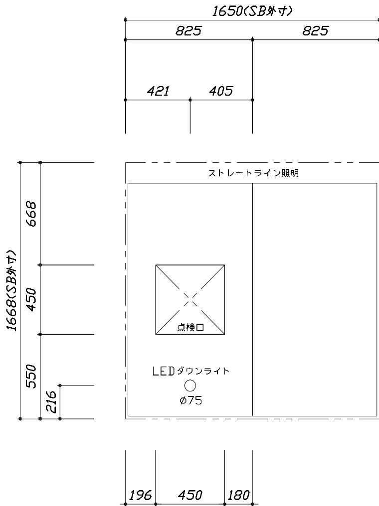
<天井伏図>
