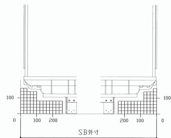
E矢視
