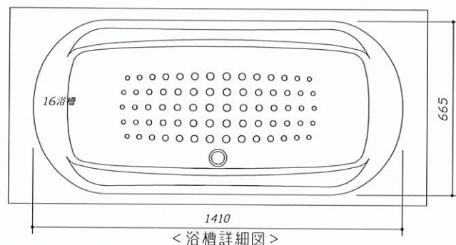
<浴槽詳細図>
