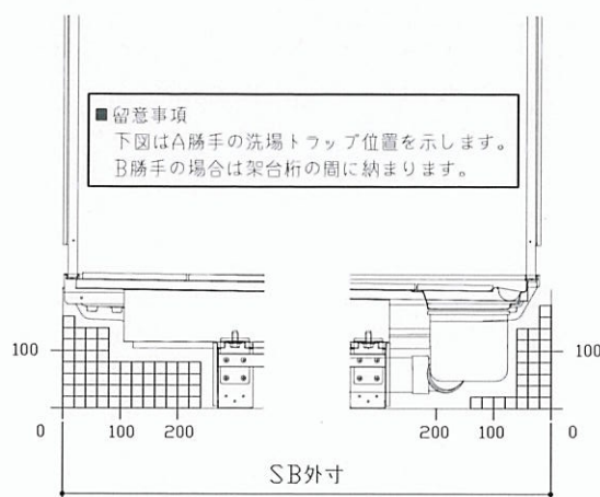
C矢視
