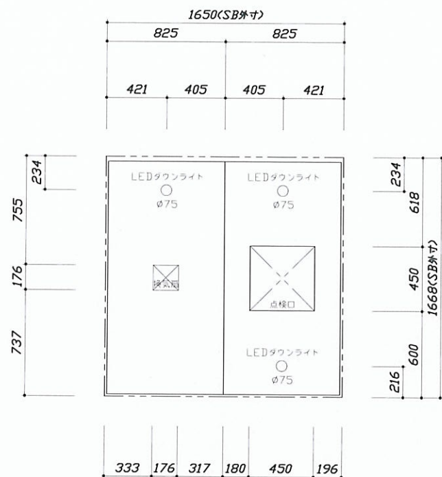
<天井伏図>
