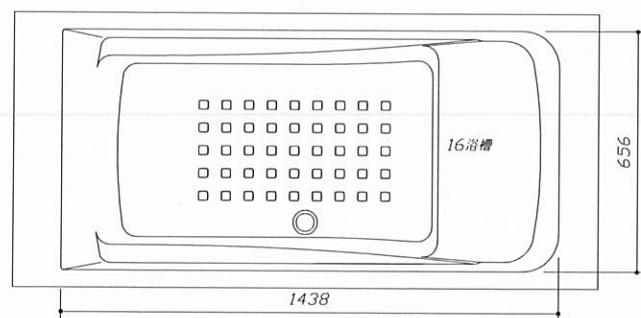
<浴槽詳細図>
