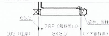
〈参考寸法図〉
