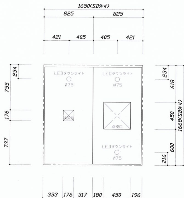
<天井伏図>
