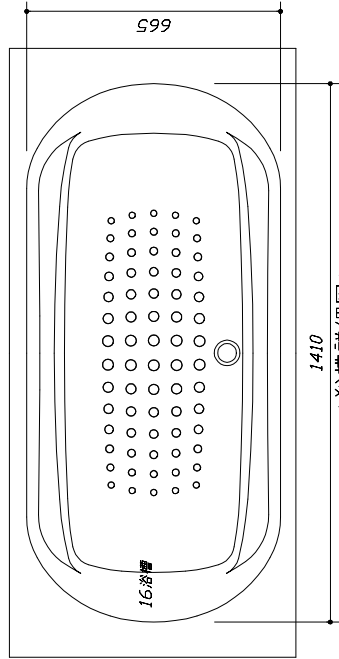
< 浴槽詳細図 >
