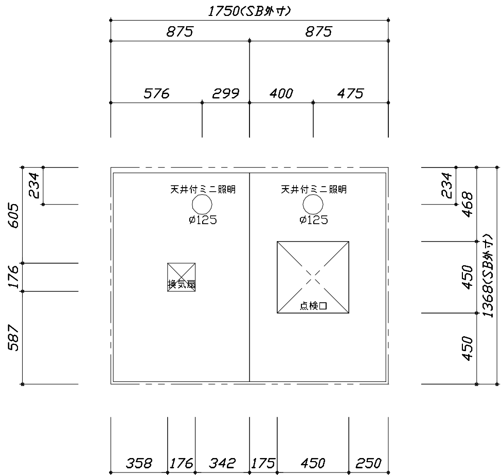
< 天井伏図 >
