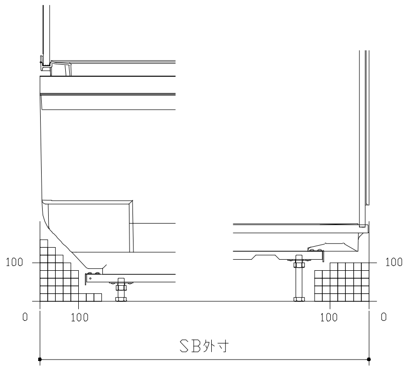
A矢視
