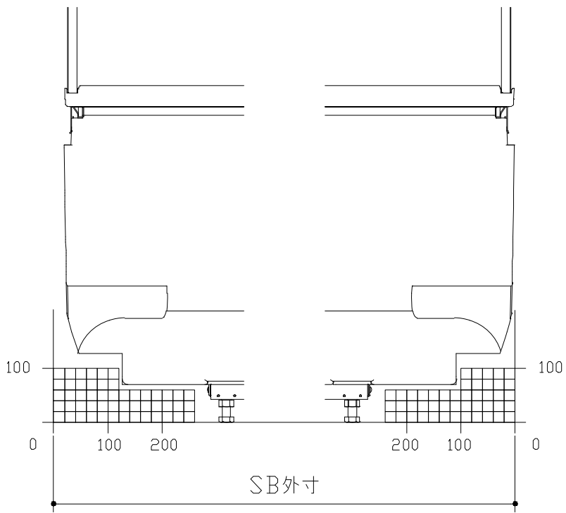
E矢視
