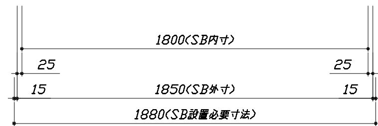
< 平面図 >
