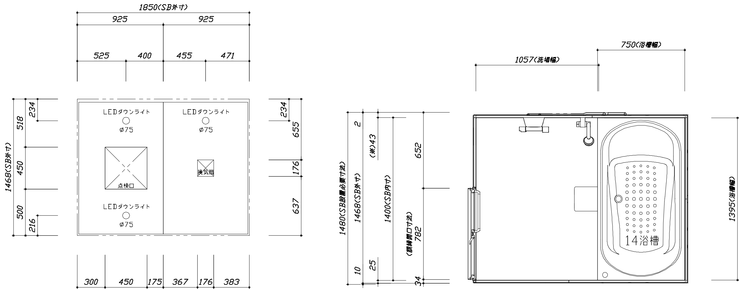
< 天井伏図 >
