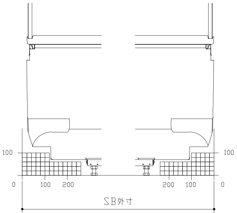
E矢視
