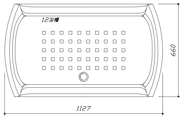
< 浴槽詳細図 >
