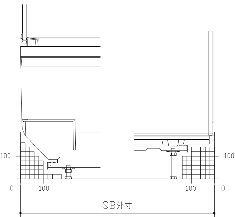
A矢視
