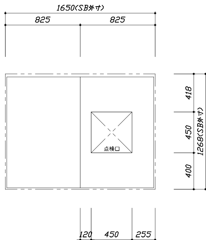
<天井伏図>
