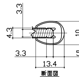
断面図
