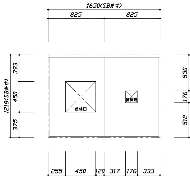
<天井伏図>
