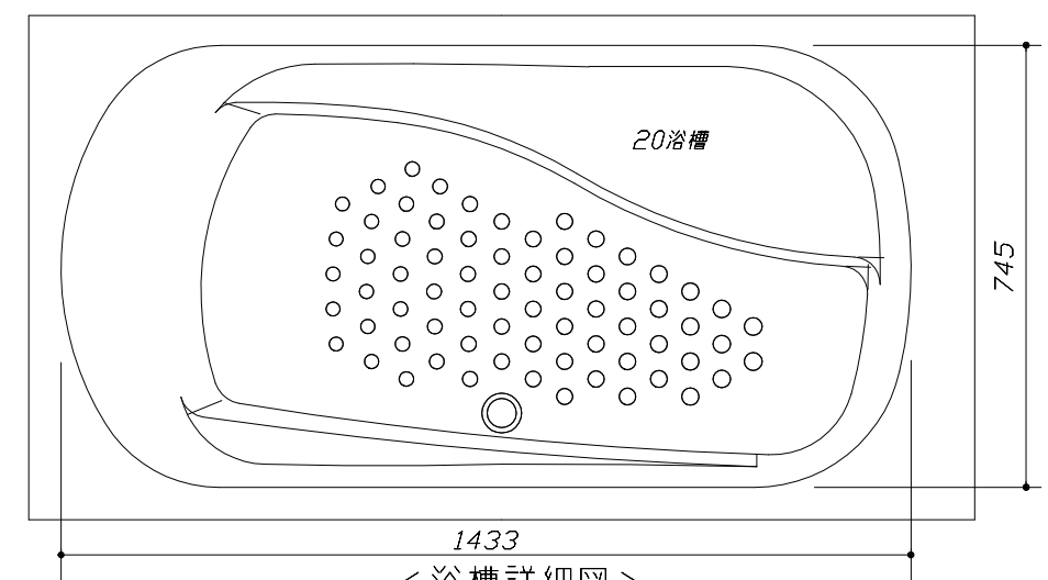
<浴槽詳細図>
