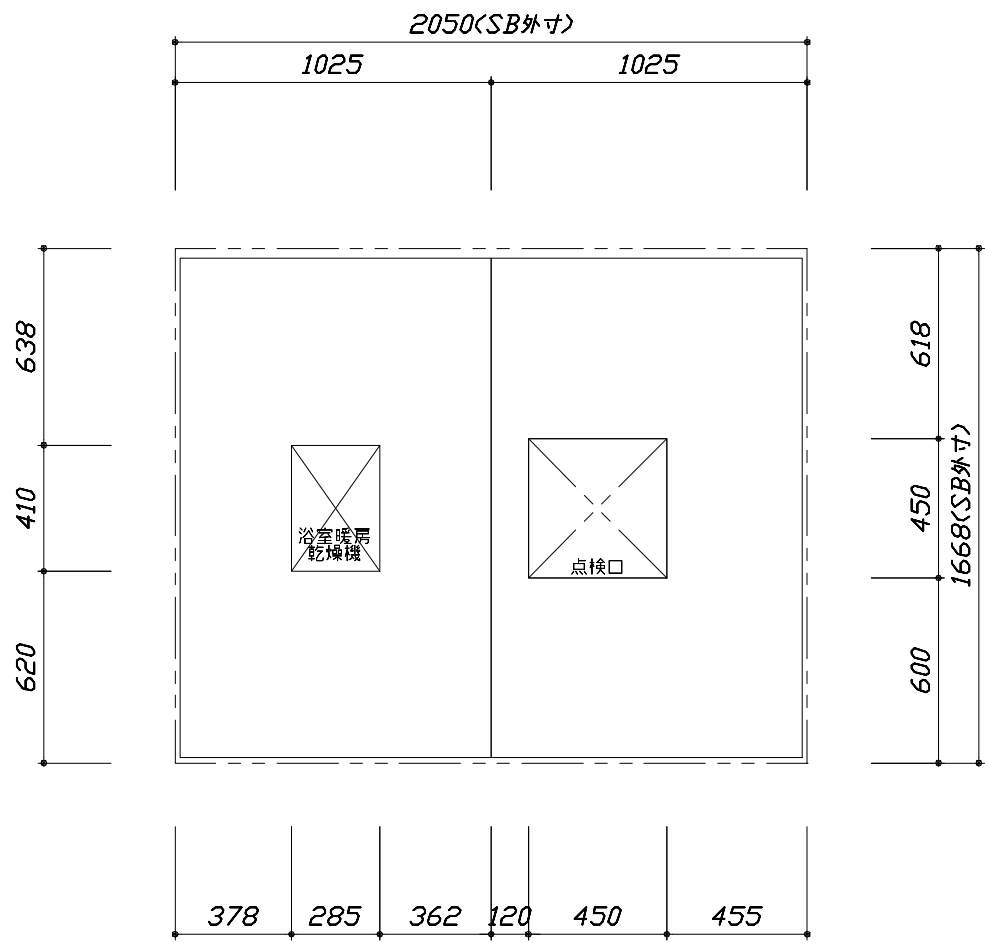
< 天井伏図 >
