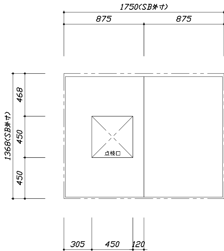
< 天井伏図 >
