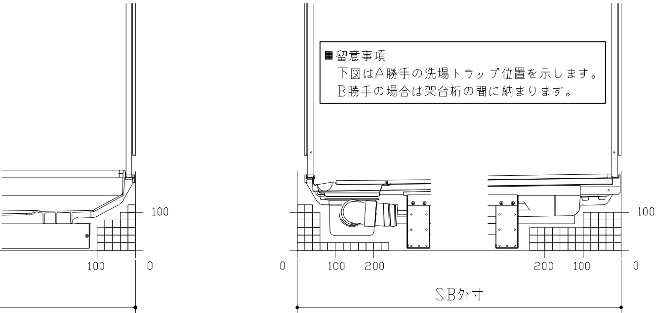
D矢視
